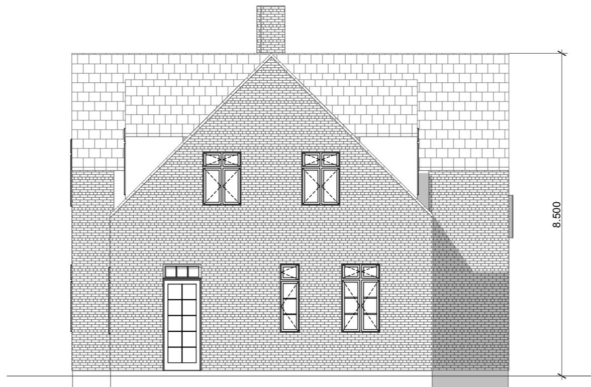
Øst Facade
