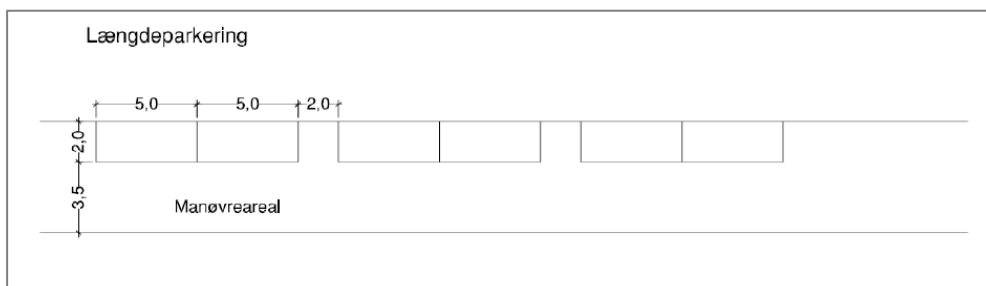
Figur 8: Vejledende længder for længdeparkeringspladser (håndbogen for Parkering og standsning i byer, jan. 2018 - fremsat)
