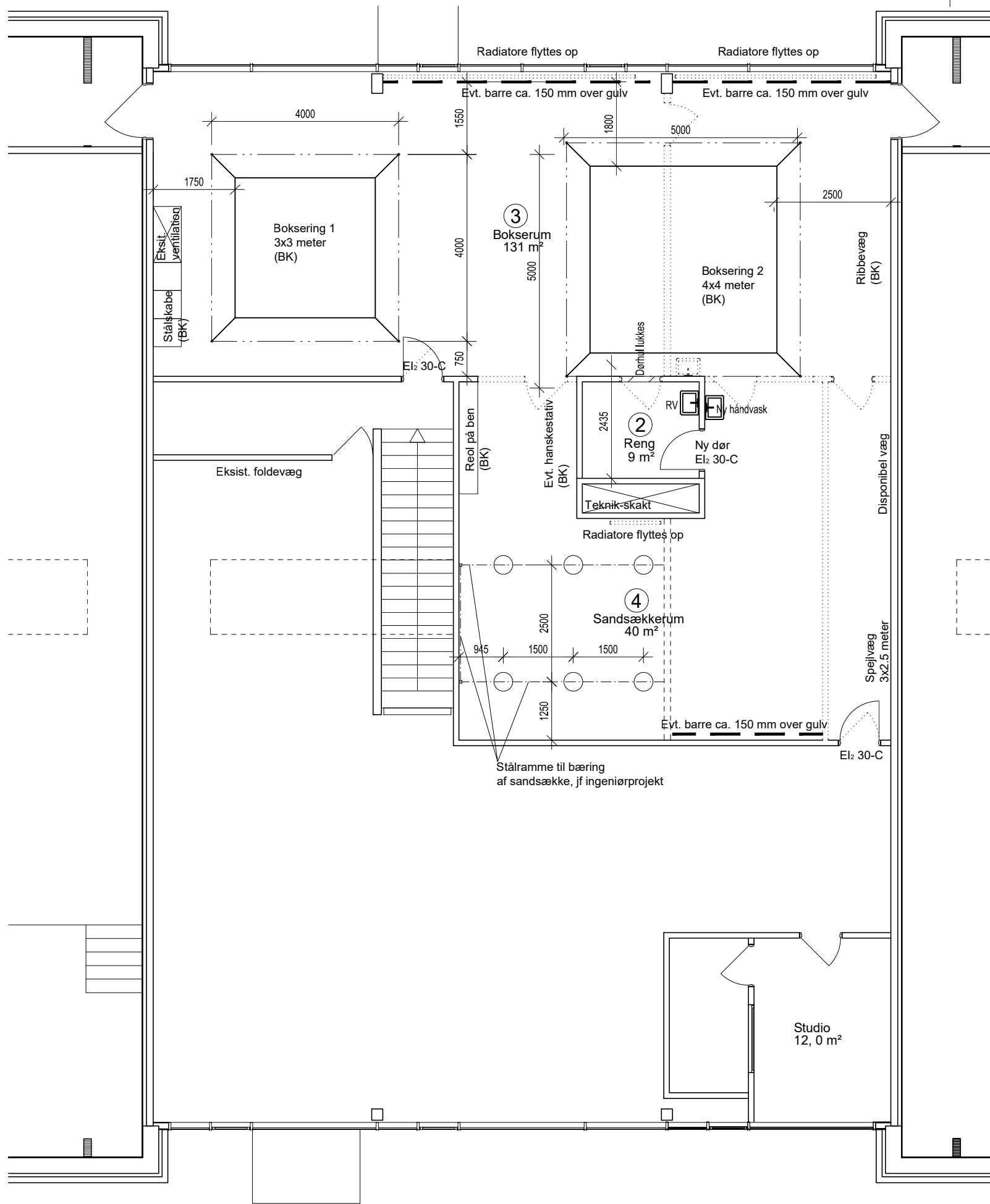
1. salsplan
