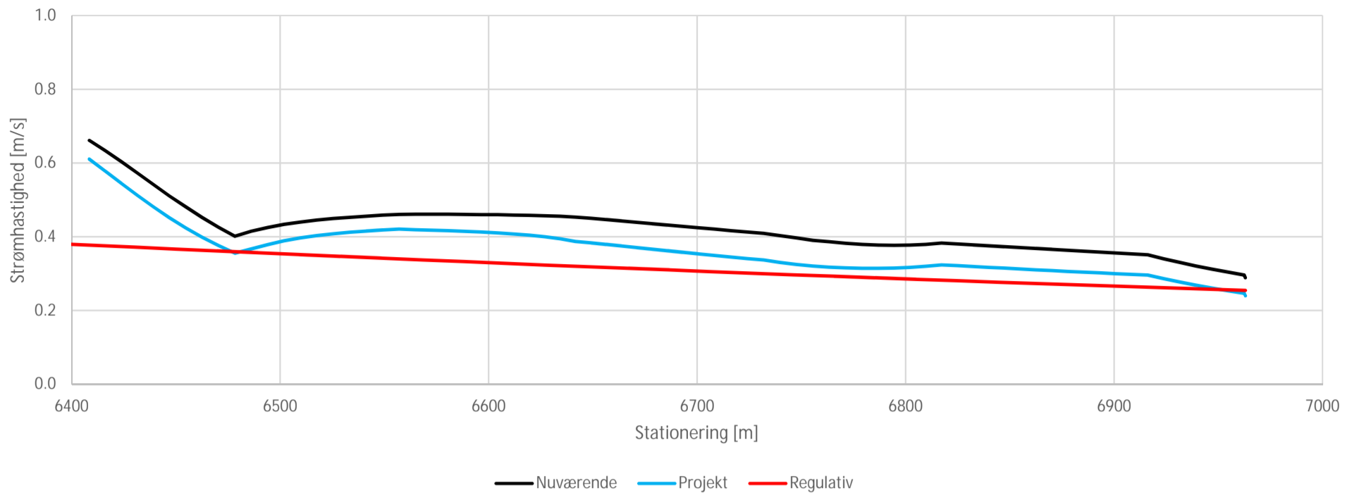
Bilag 6.3 Strømhastighed ved medianmaksimumafstrømning Mølleåen
