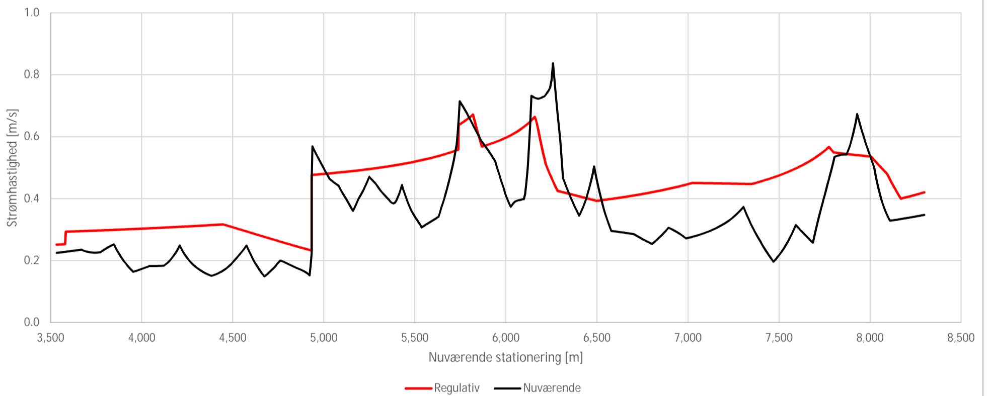
Strømhastighed ved medianmaksimumafstrømning Vigersdal Å
