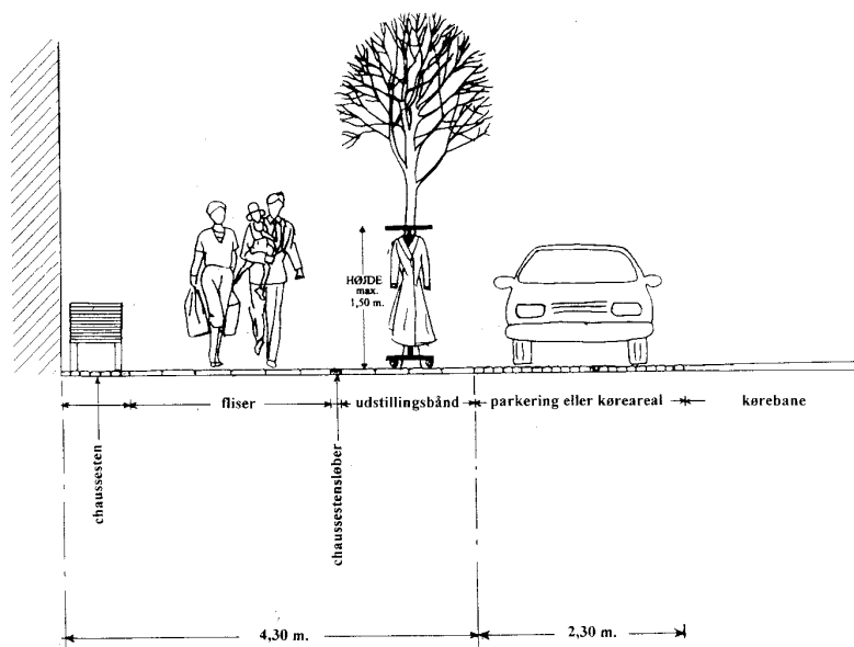
Tværsnit ved 4,30 m. fortovsbredde.
